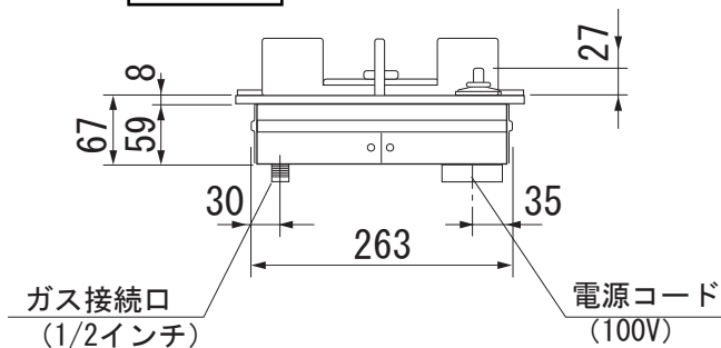
正面図
